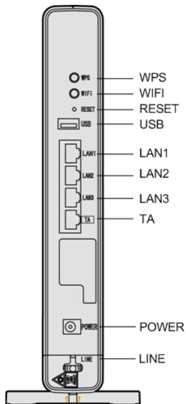
図 1-2 ZXHN F660T 背面ポートとボタン
